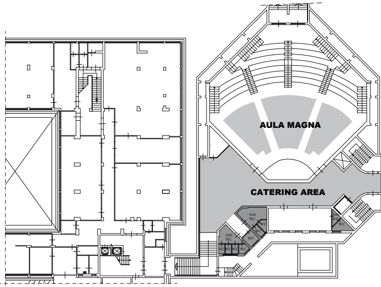
Building E (Edificio 13)_ Aula Magna
